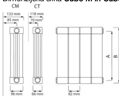
Dimenzijska slika Cubo M in Cubo T:
