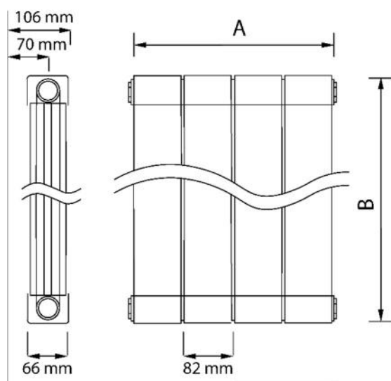
Dimenzijska slika Smart :
